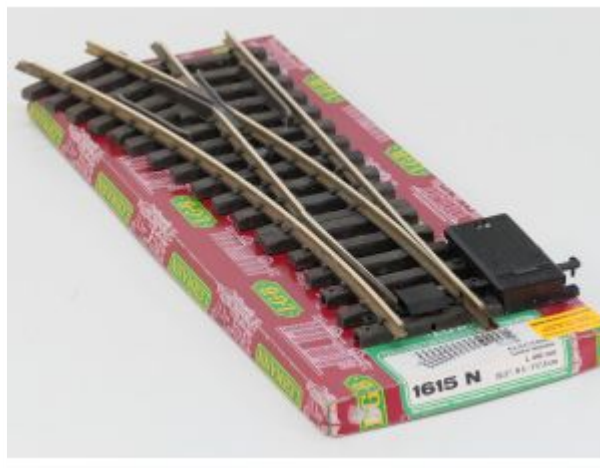
LGB 16150 Elektr.Weiche,Links.R3,22.5Grad
