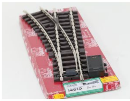
LGB 14615 Elektrische Weiche, Vernickelt, Links, R3, 22,5°
