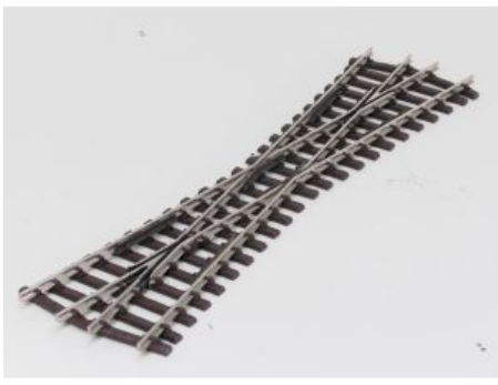
THIEL 2511 Kreuzungen 15° Nickel. Buiten Gebruikt
