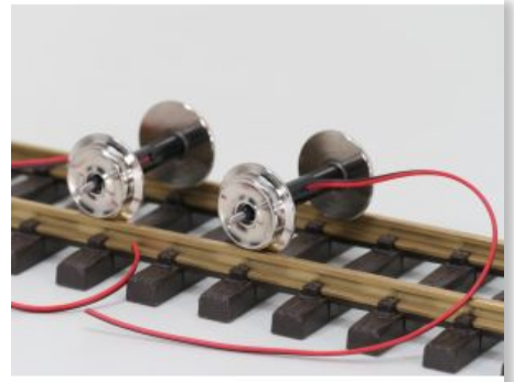
GS Kugellager-Radsatz, Stomabnahme, 2 St, Technisch Zoals LGB 67403 / Piko 36167, Ø 25 Mm Bij ons: € 39,95
