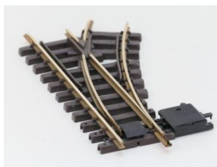
LGB 12000 Handweiche Rechts, R1, 30 Grad
