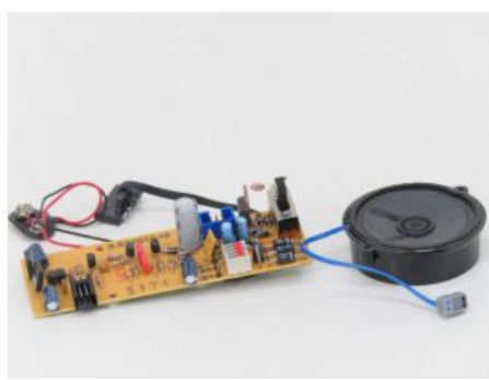
LGB 20604 Sound Module
