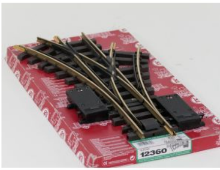
LGB 12360 Elektrische Dreiwegweiche, R1, 30 Grad
