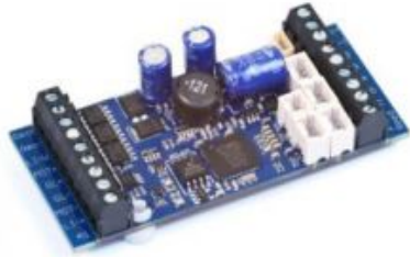
Massoth 8210570 eMOTION XLS Emma, Soundprojekt für LGB 22222 Emma
