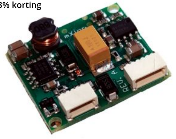
Mxion 8000 SX6 16 Bit Sound, 640 Sek. Speicher, 40 Einzelgeräusche SUSI Soundmodul Mit Puffer 3W Mit KABELN
