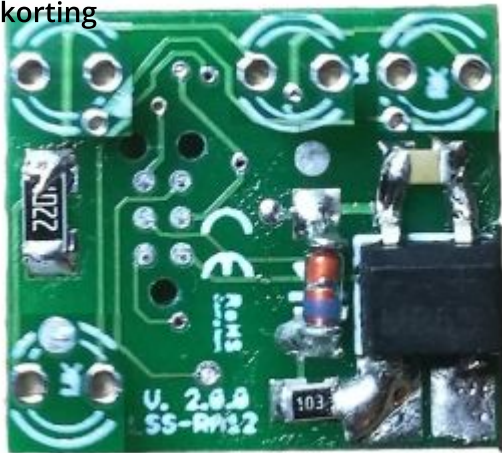
Mxion 4601 LSS 3 Kanal Signaldecoderplatine
