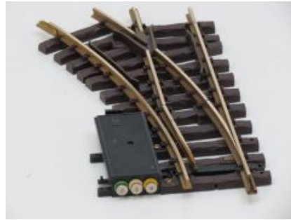
LGB 1215 Elektr.Weiche li.,R1,30Grad, (oud model)
